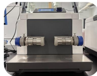
【メカノケミカル有機合成装置例】
